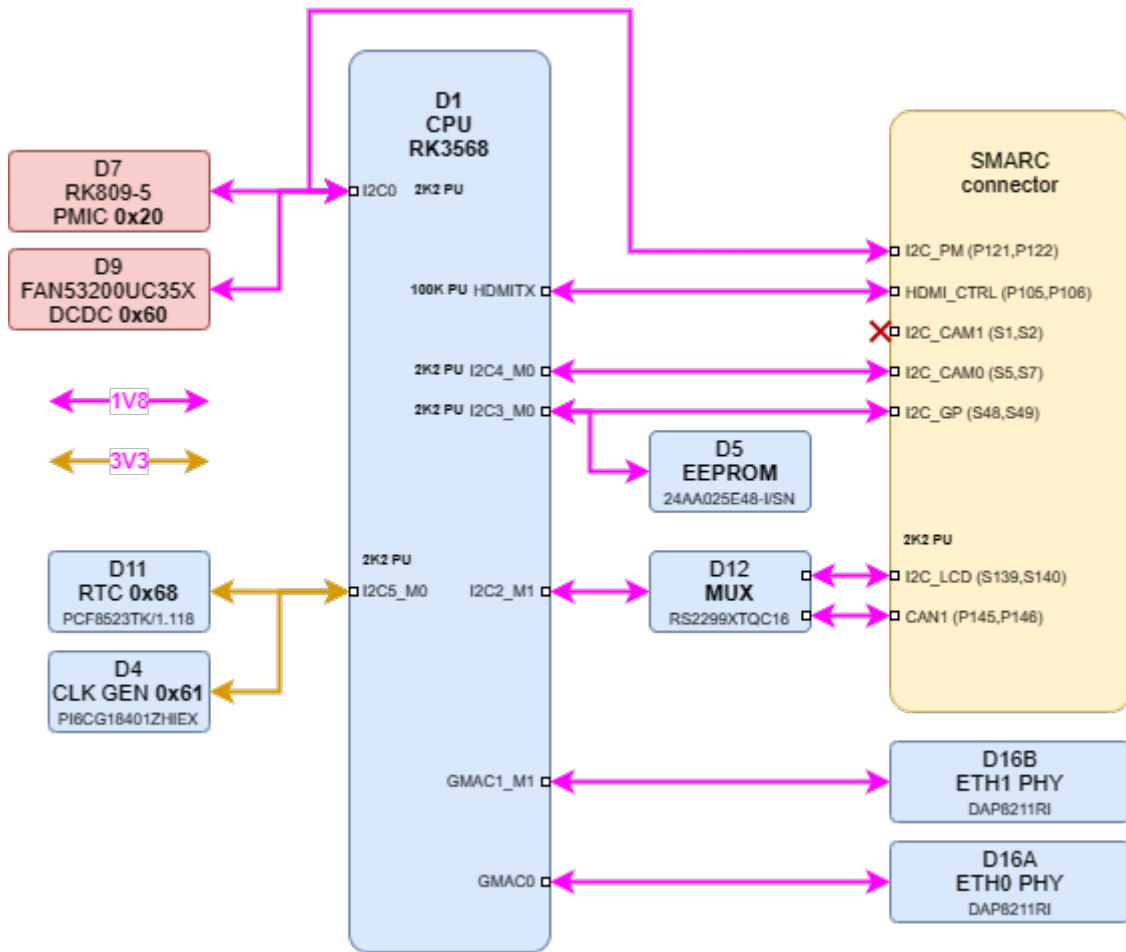
Рисунок 6: I2C интерфейс
