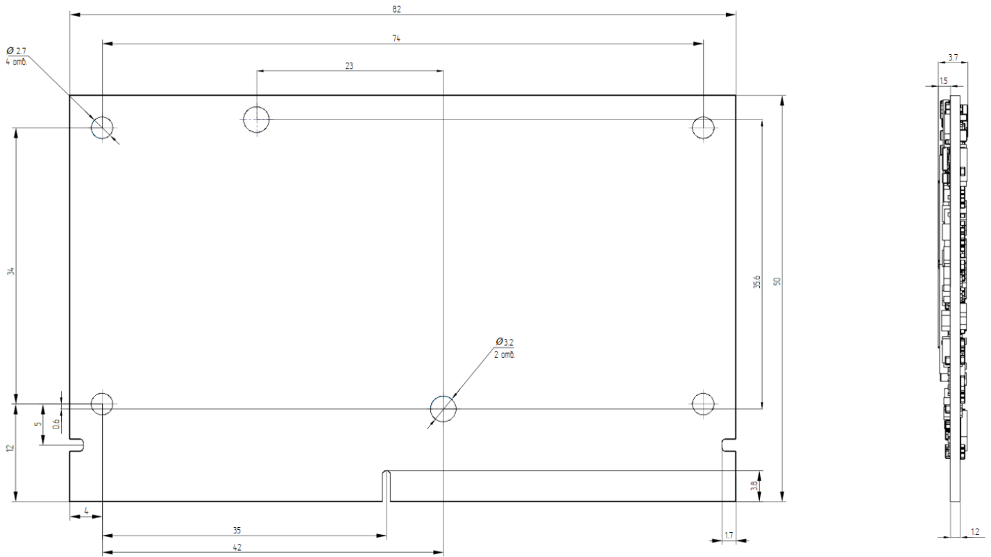
Рисунок 2: Габаритные размеры
