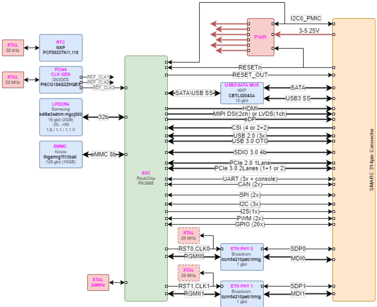
Структурная схема модуля
