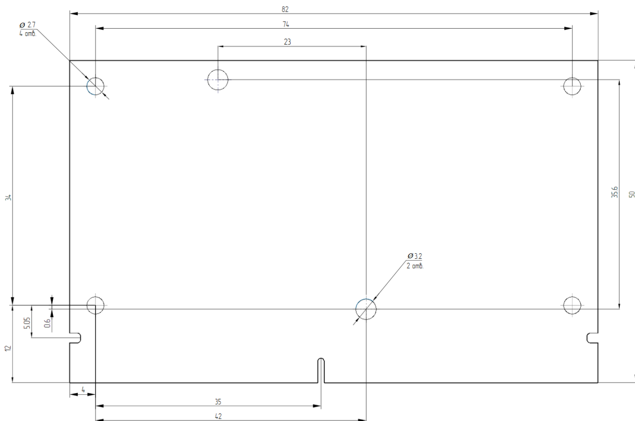
Габаритные размеры
